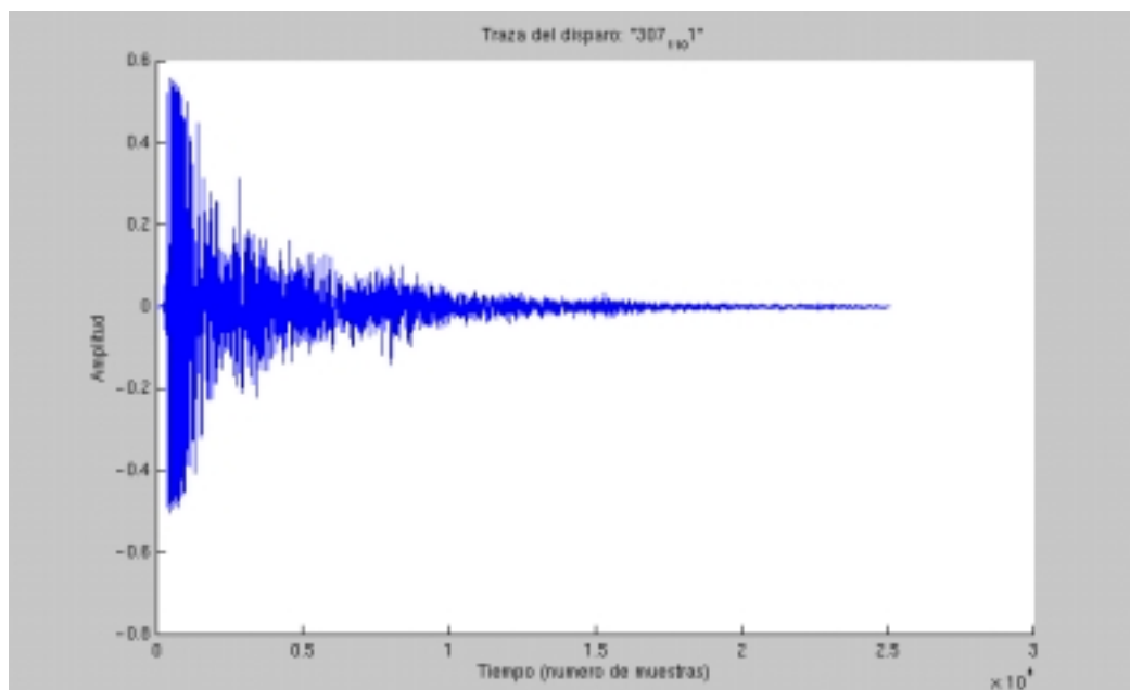
Figura 4.13. Trazo de la señal de disparo emitido por una escopeta en la galería interior.
