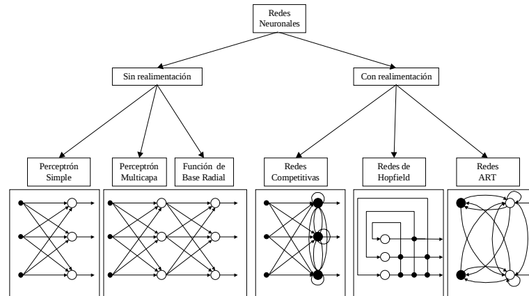
Figura 7.9. Una taxonomía de RNA.
