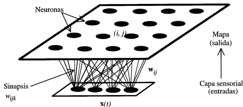
Figura 7.12. Arquitectura de SOM.
