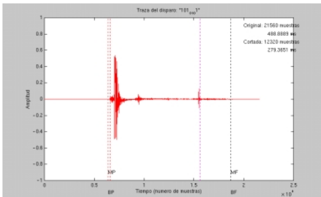
Figura 4.32. Taza de la señal de un disparo de una pistola en la galería interior.
