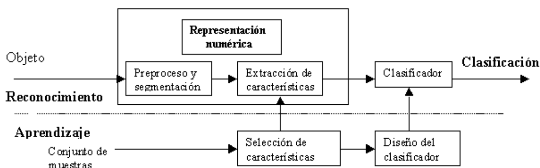
Figura 6.1. Proceso de clasificación.
