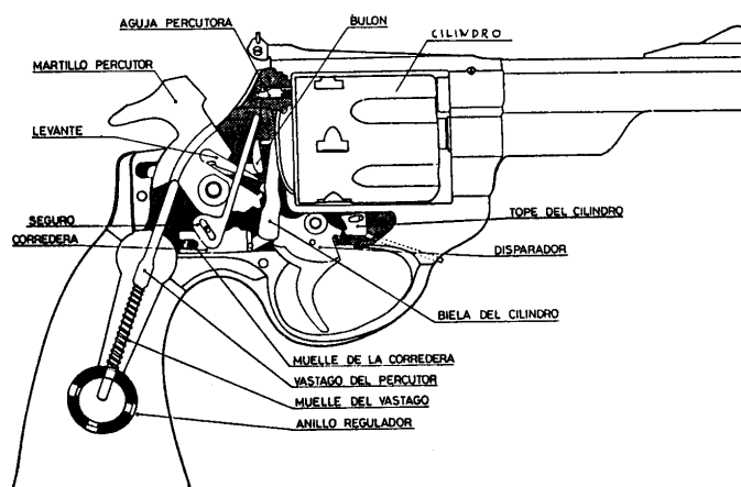
Figura 1.18. Esquema del revólver.
