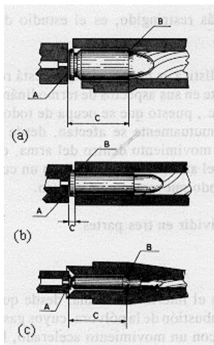
Figura 1.1. a) En el cartucho cilíndrico de ranura, la boca de la vaina. b) En el cartucho cilíndrico de pestaña, la parte anterior de la pestaña del culote. c) En el cartucho de vaina abotellada, la gola.
