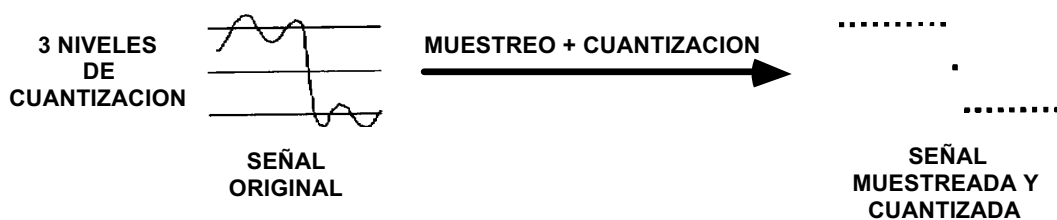
Figura 3.2. Proceso de muestreo y cuantificación.
