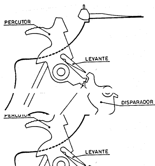
Figura 1.23. Funcionamiento en doble acción.
