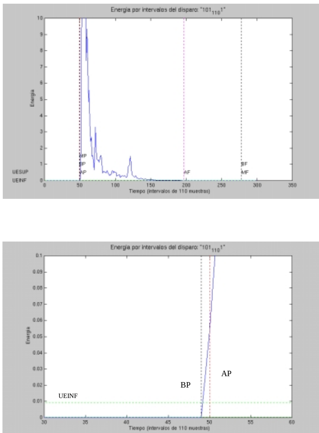
Figura 4.18. Energía de la señal por intervalos solapados a mitad para el disparo de una pistola en la galería interior y ampliación del principio de la señal.
