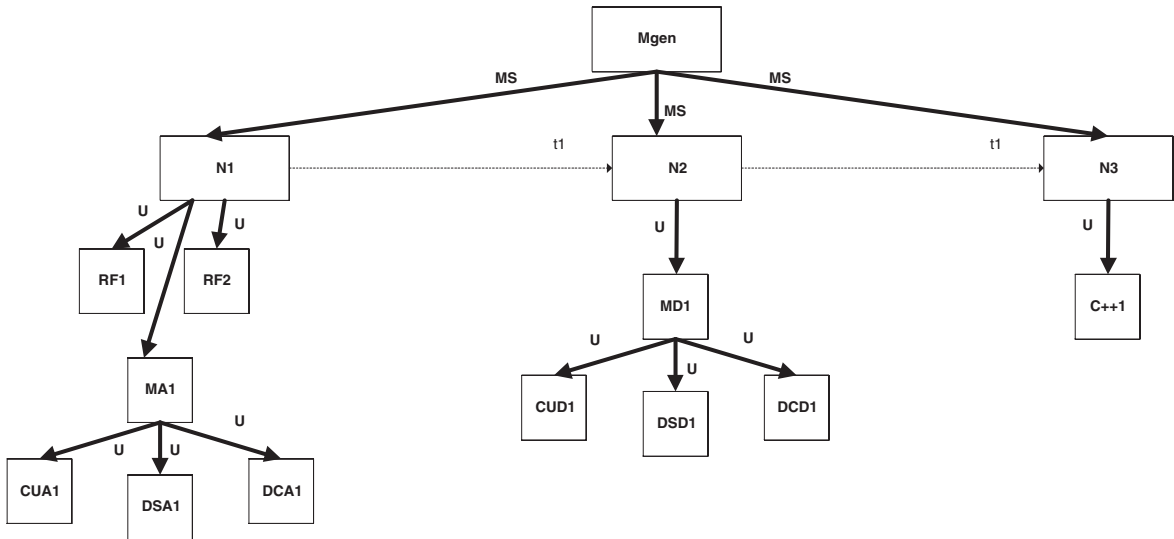
Figura 4.9: Árbol de contención parcial de M_g con respecto a Mecano_1 .
