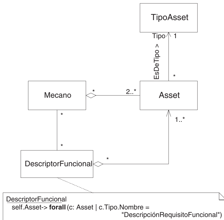
Figura 3.11: Descriptores funcionales en los mecanos.
