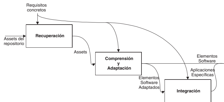
Figura 1.4: Actividades en el desarrollo con reutilización [Girardi, 1998].
